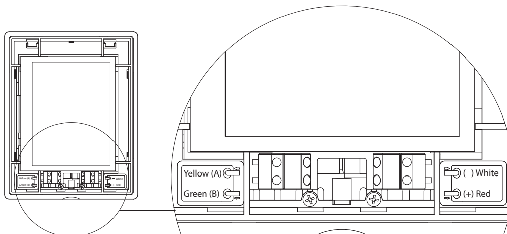
Abbildung 5.6. Anschluss des Bedienfelds
